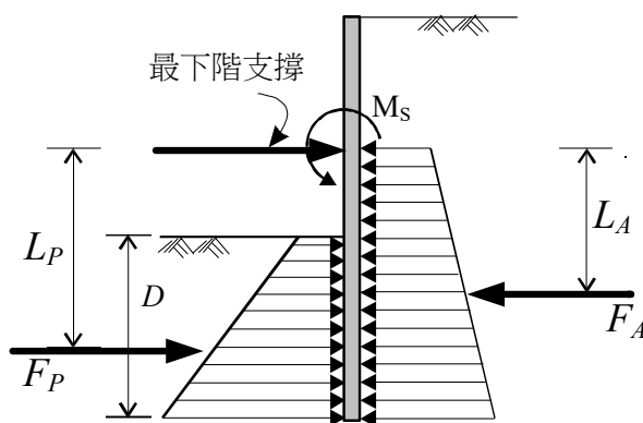
圖8.8-1 側向壓力平衡
